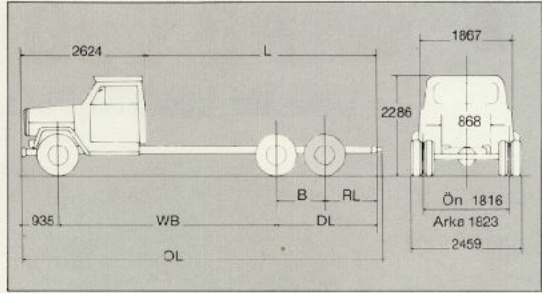
UZUNLUKLAR (mm)
